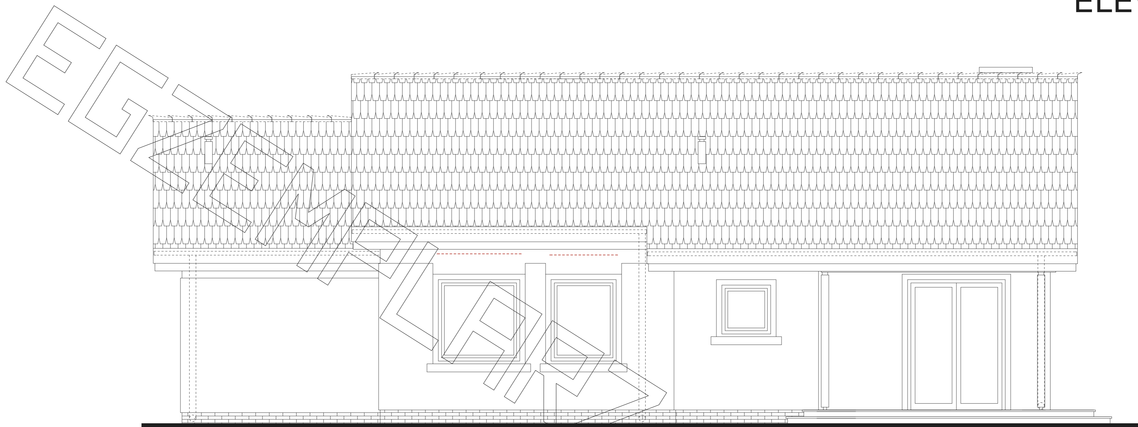
elewacja tylna
