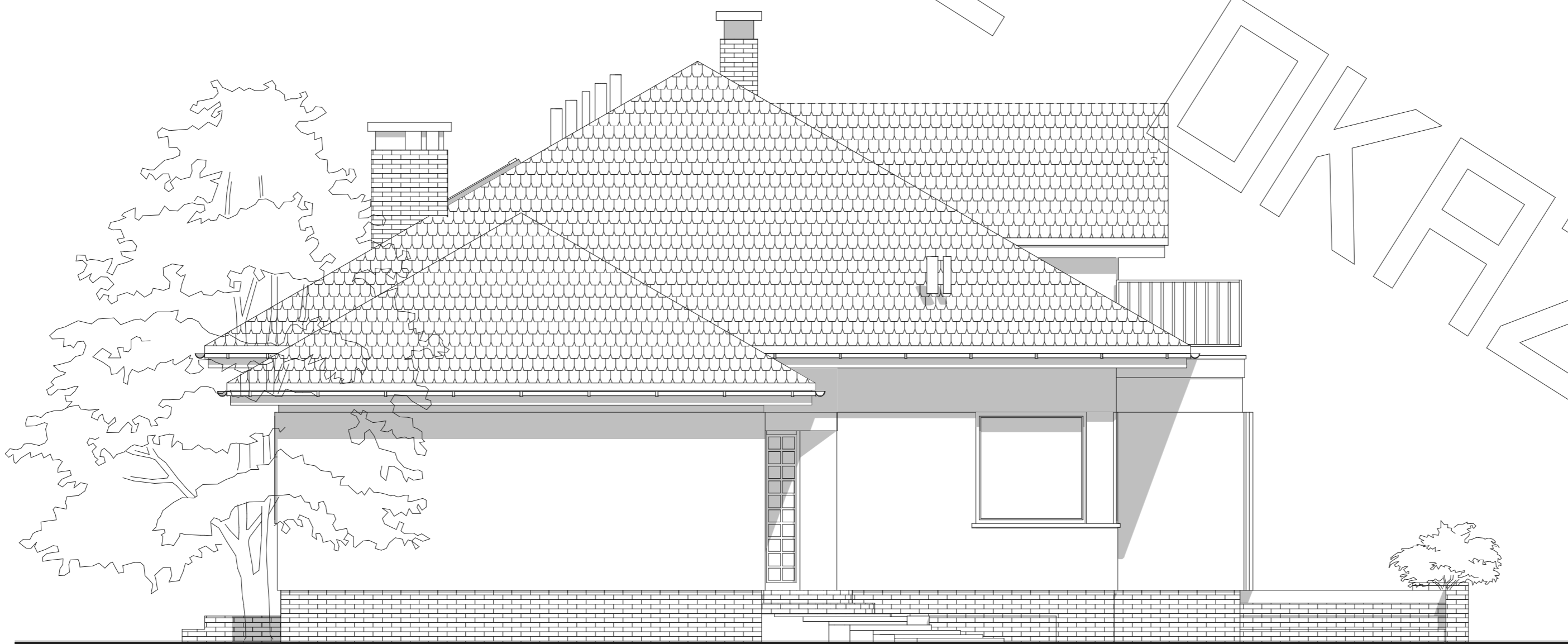
ELEWACJA BOCZNA:
