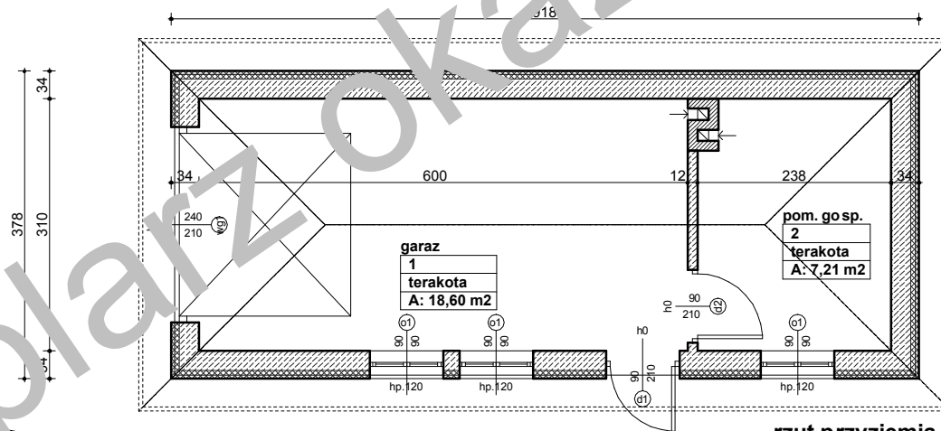
rzut przyziemia :
