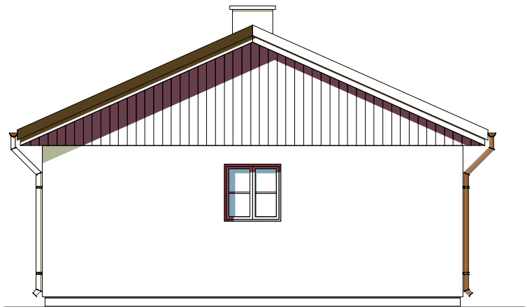
elewacja frontowa :
