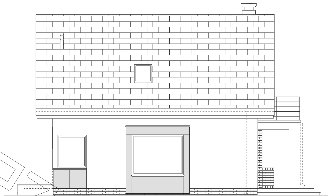
ELEWACJA BOCZNA :
