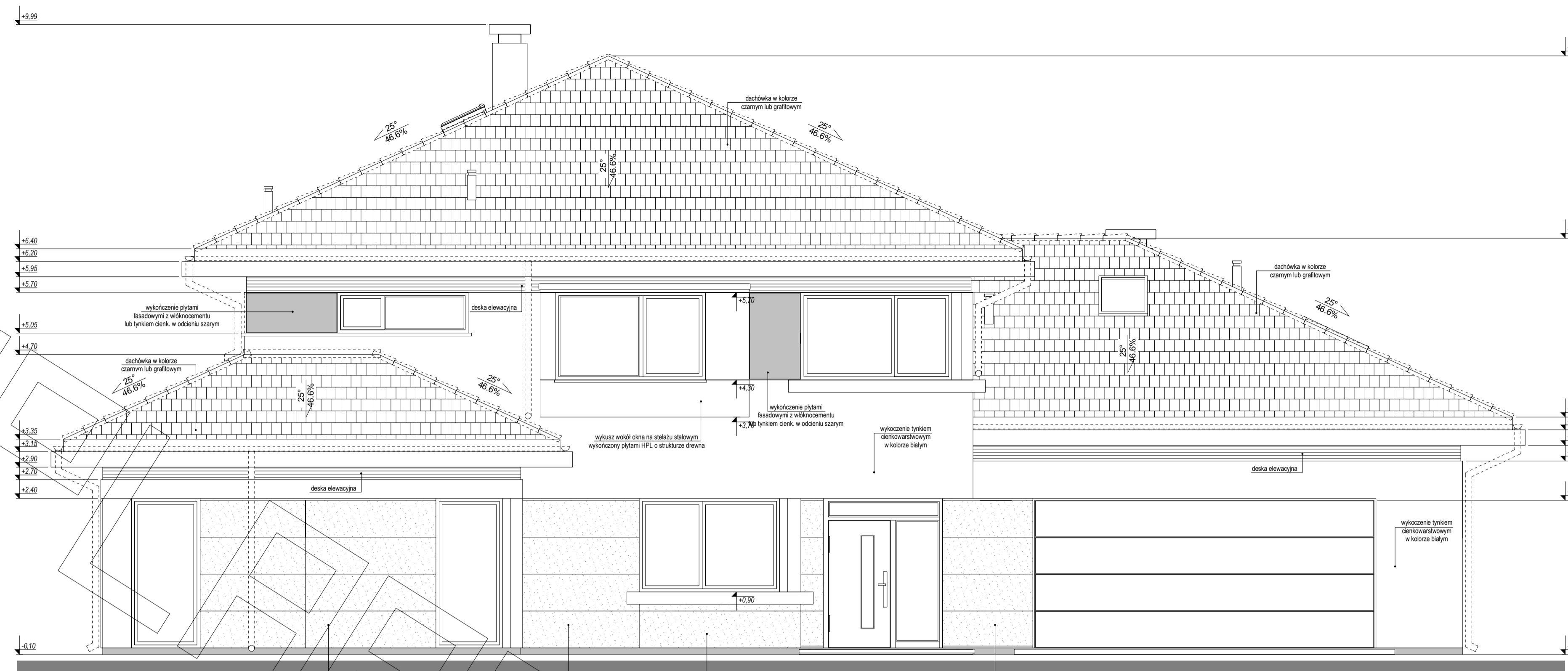
elewacja frontowa : północna
