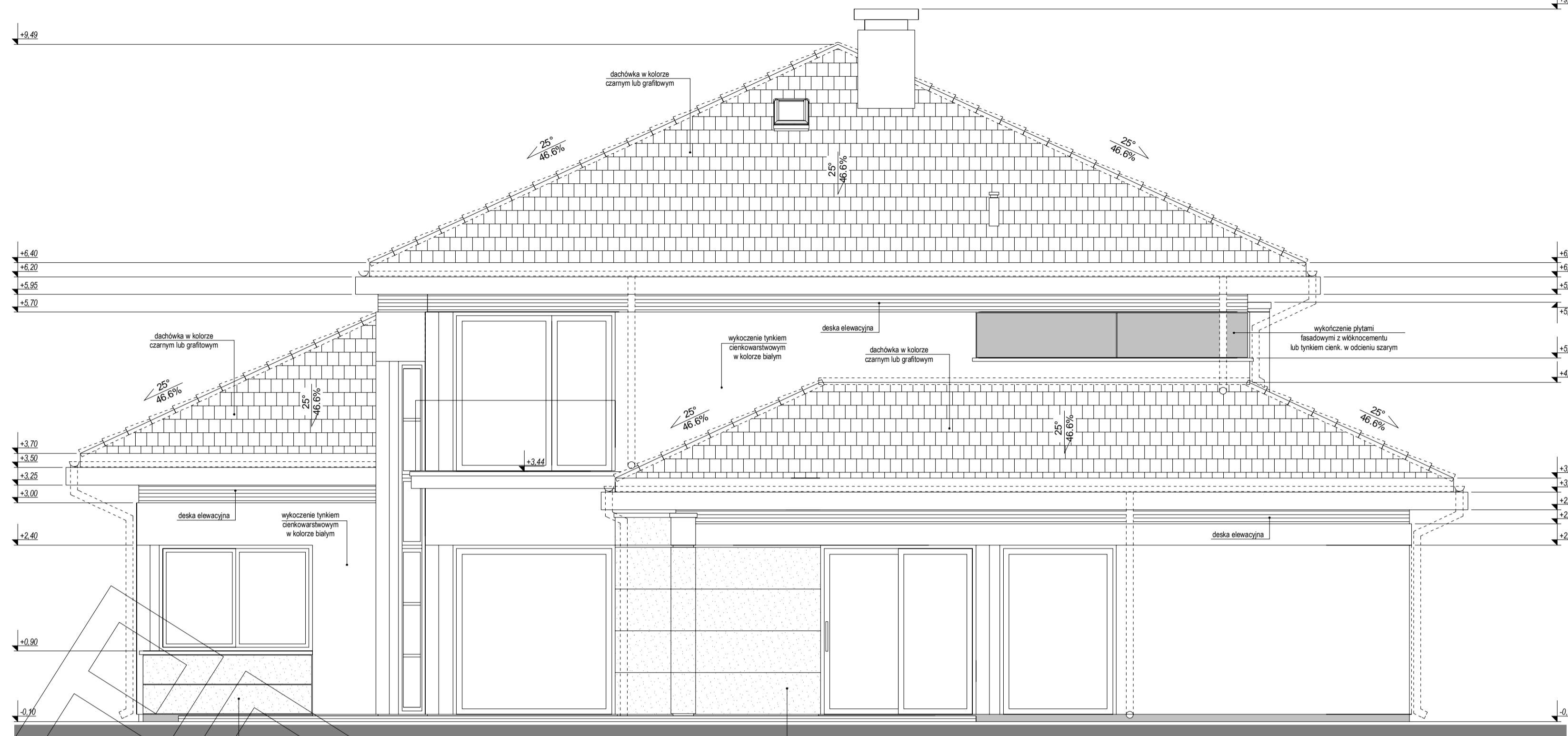
elewacja boczna : wschodnia
