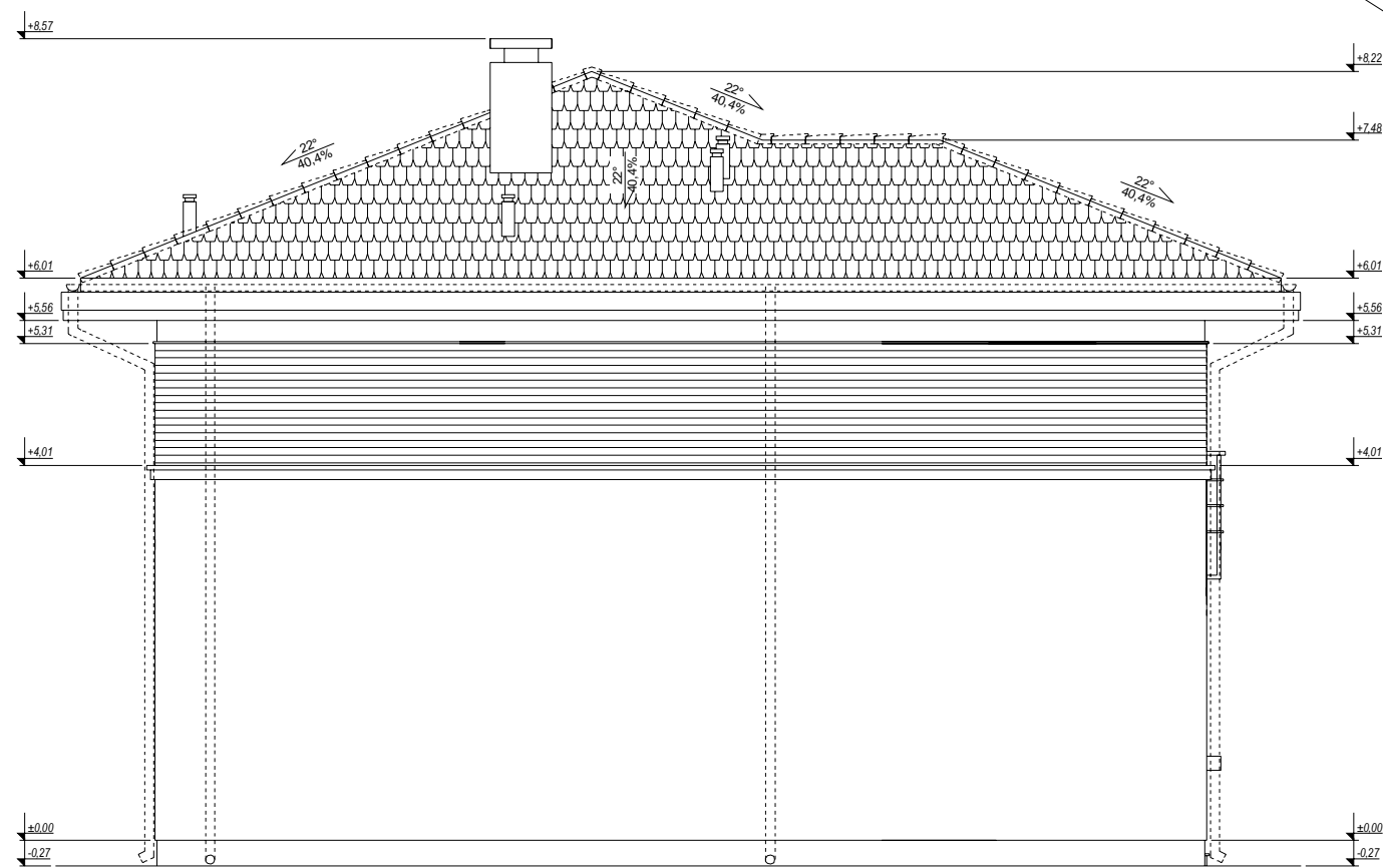
elevacja boczna :
