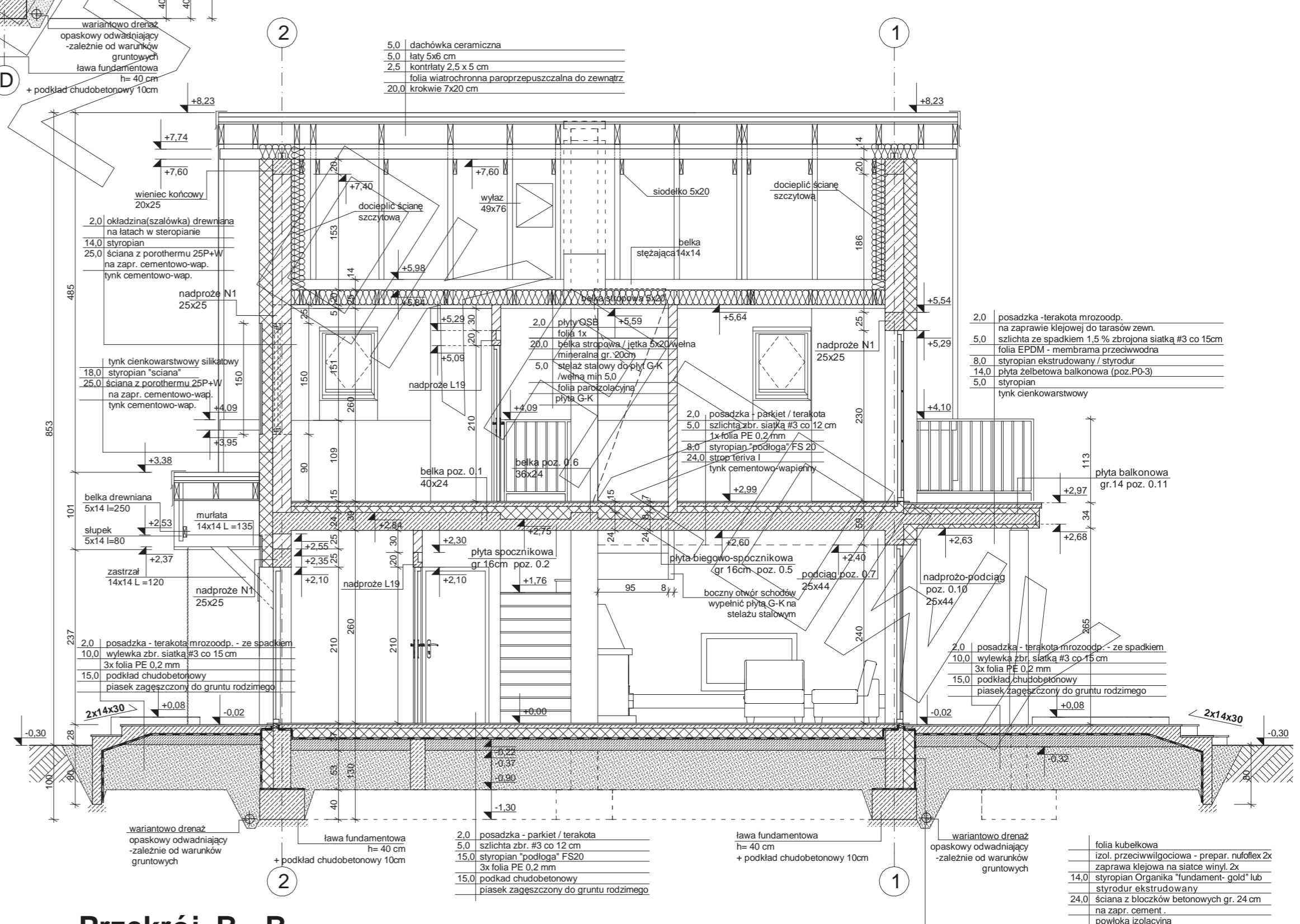
Przekrój B - B
