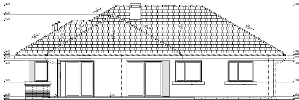
elewacja boczna :
