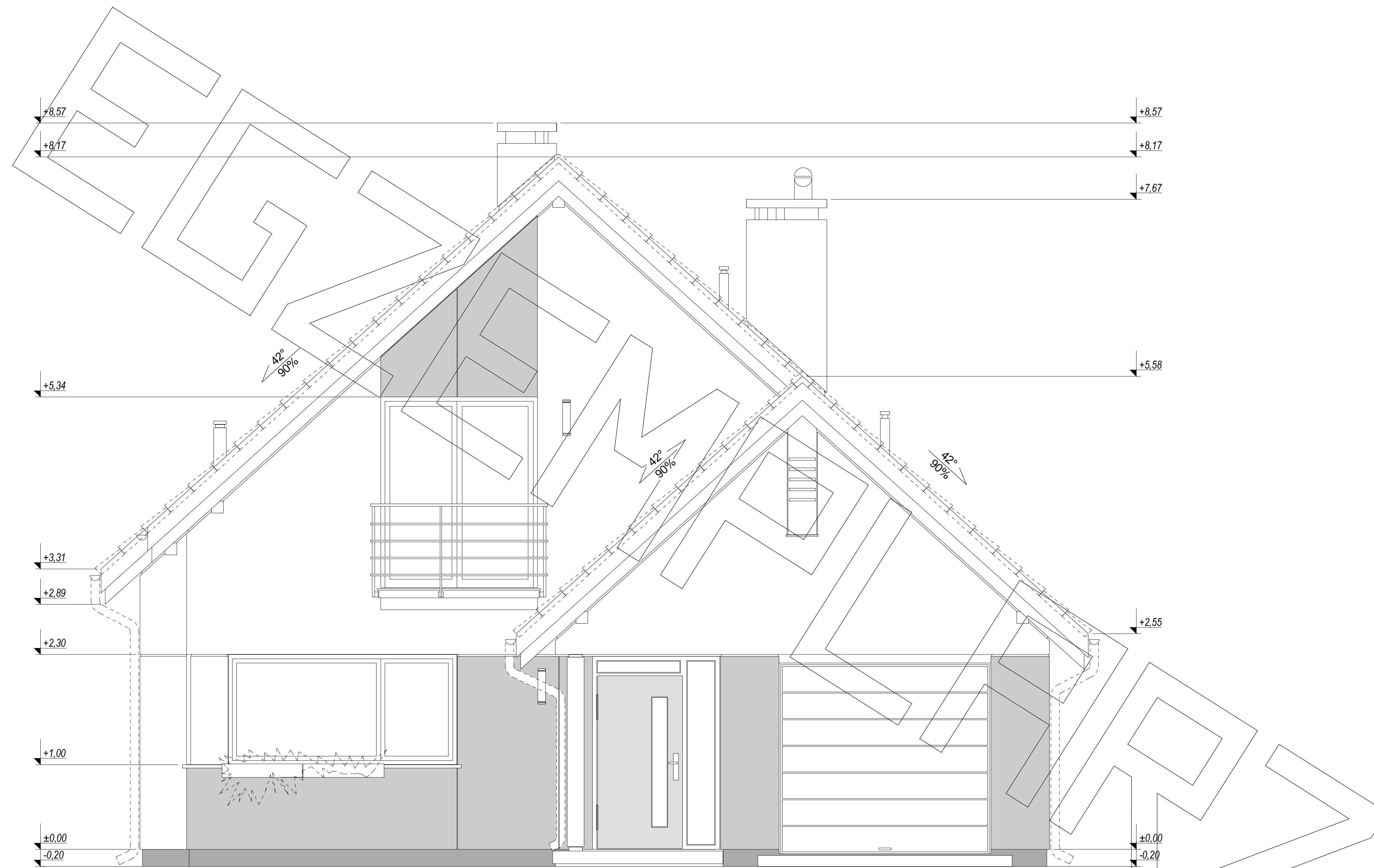
elewacja frontowa :
