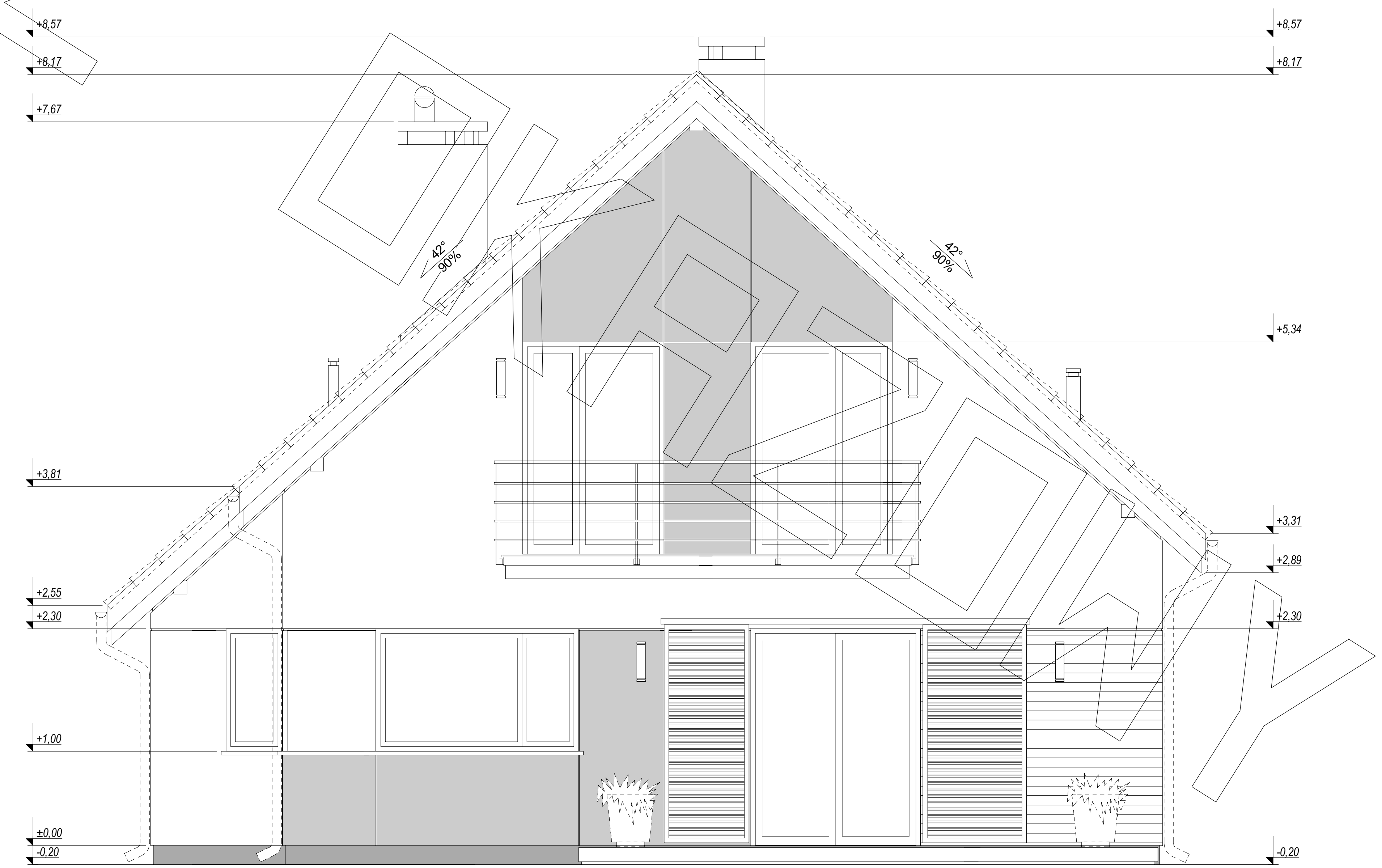
elewacja ogrodowa :
