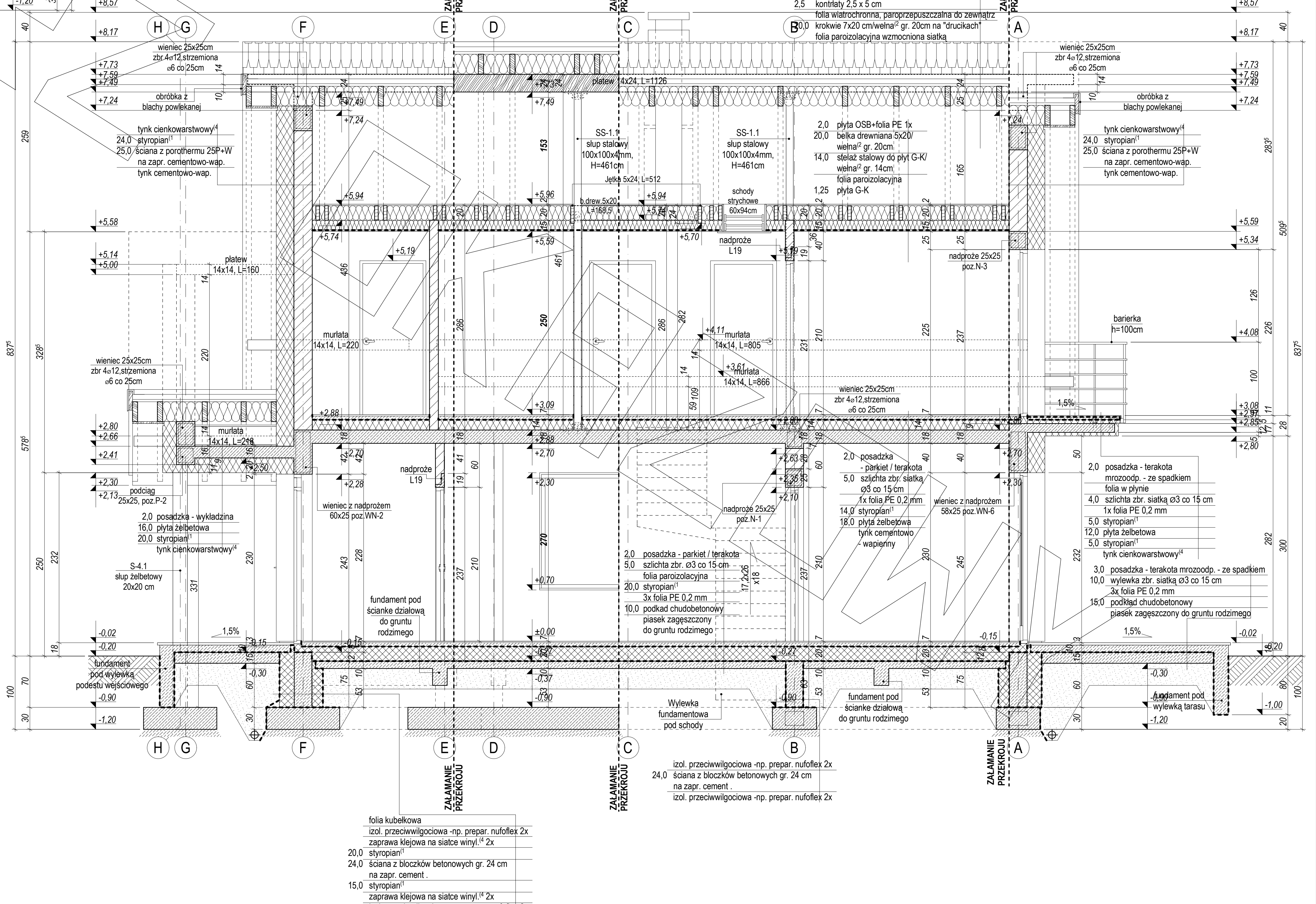
PRZEKRÓJ B - B
