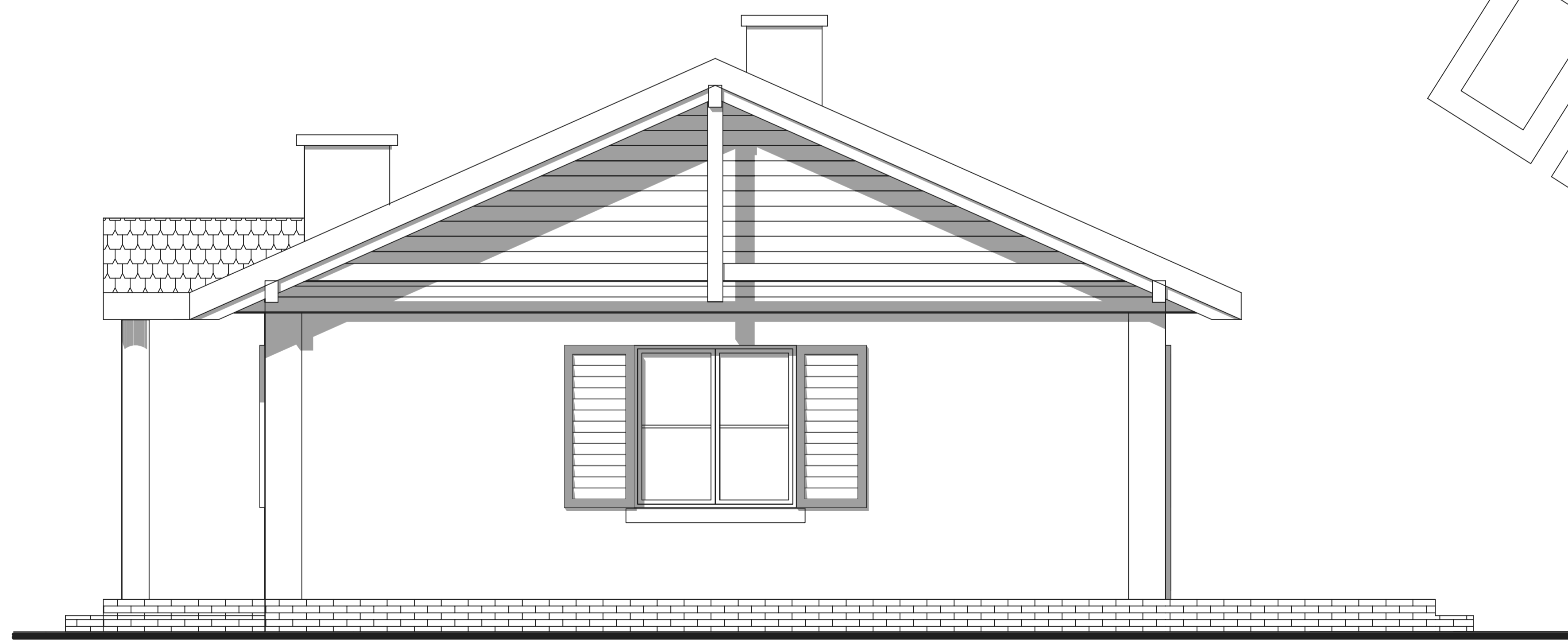
elewacja boczna :
