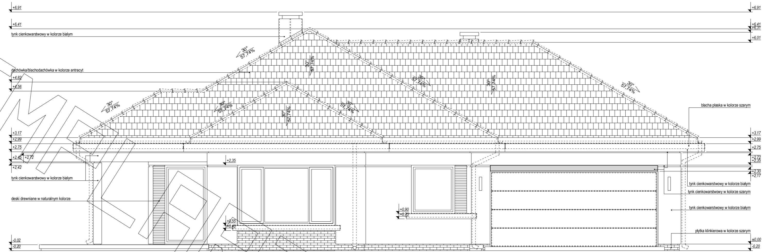
ELEWACJA FRONTOWA:
