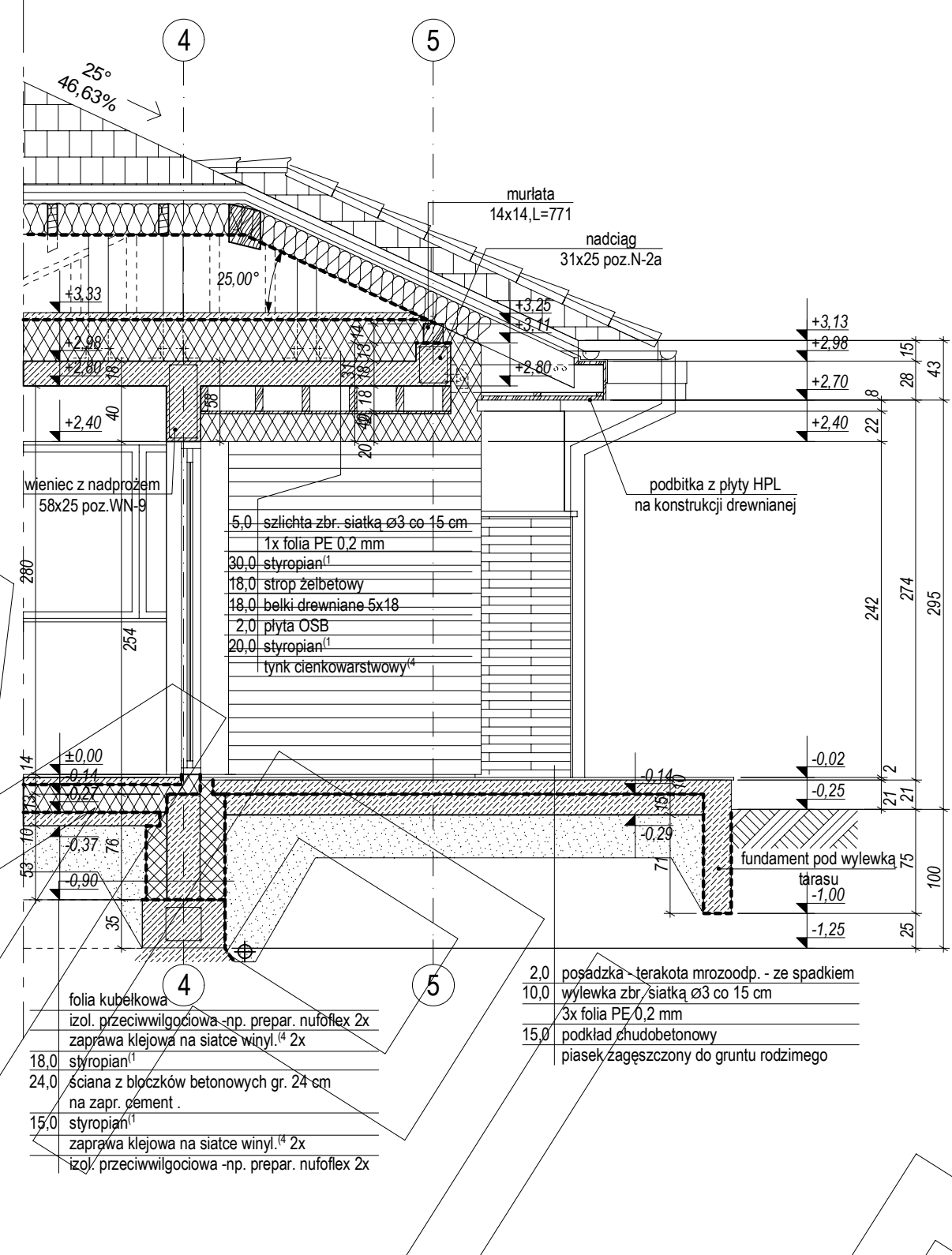
PRZEKRÓJ A1-A1
