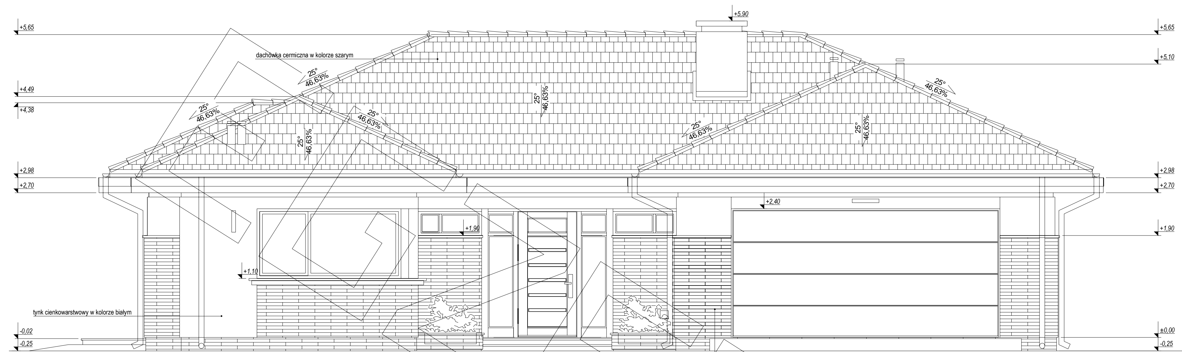
ELEWACJA FRONTOWA
