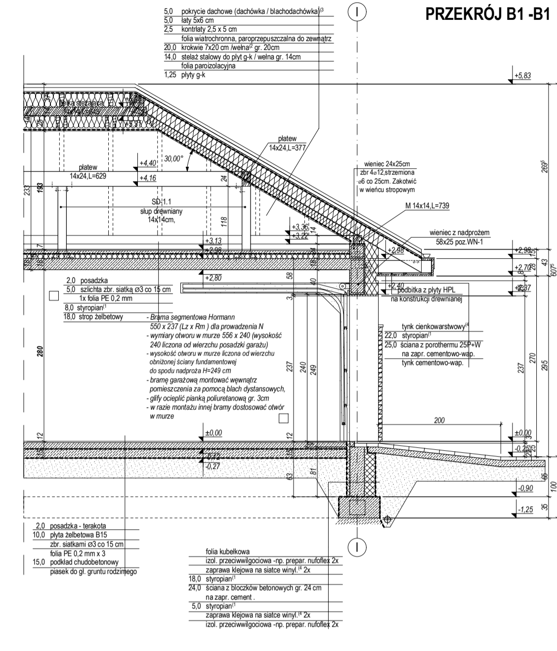
PRZEKRÓJ B1-B1
