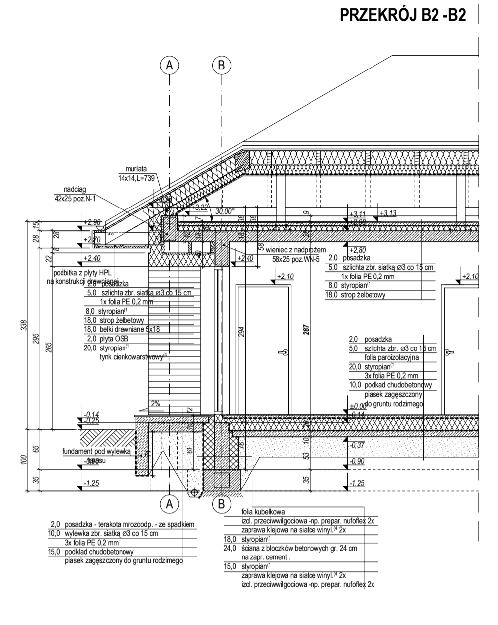
PRZEKRÓJ B2-B2
