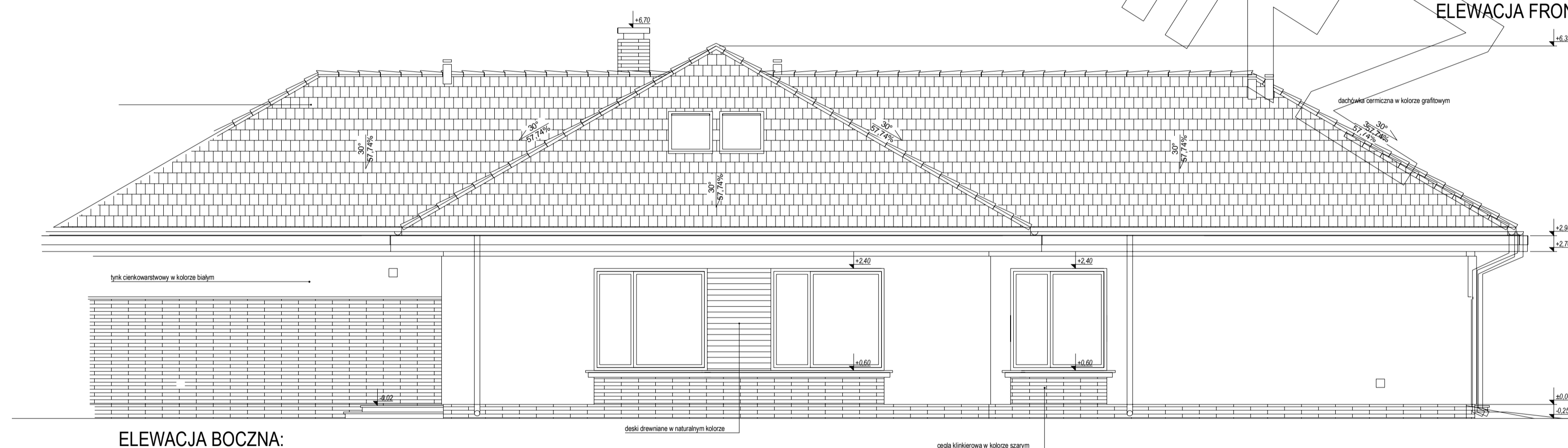
ELEWACJA BOCZNA:
