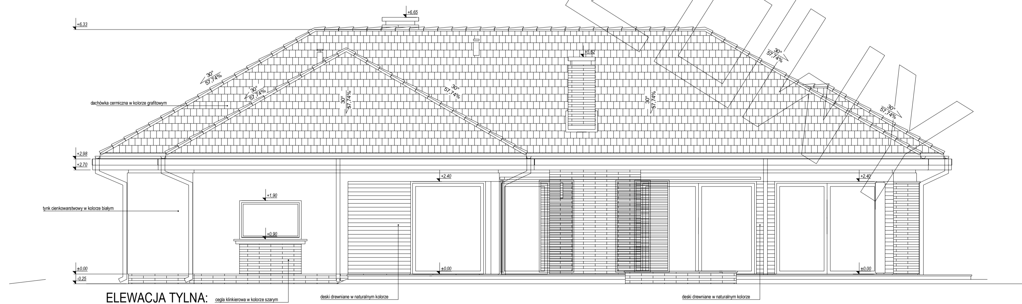
ELEWACJA TYLNA:
