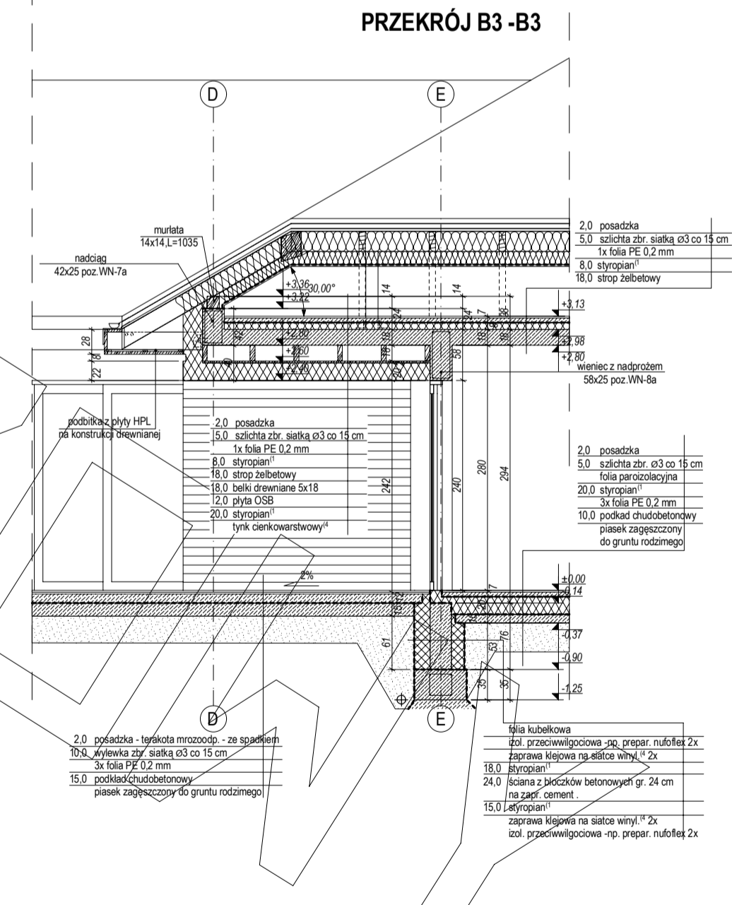
PRZEKRÓJ B3-B3
