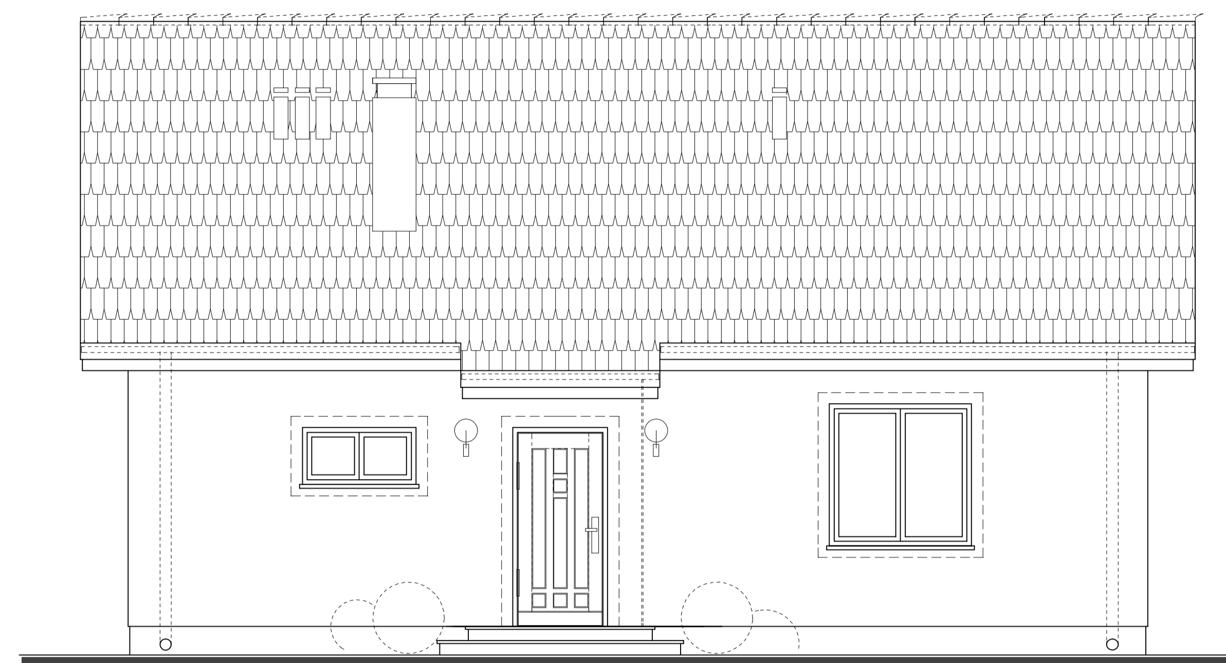
Elewacja frontowa
