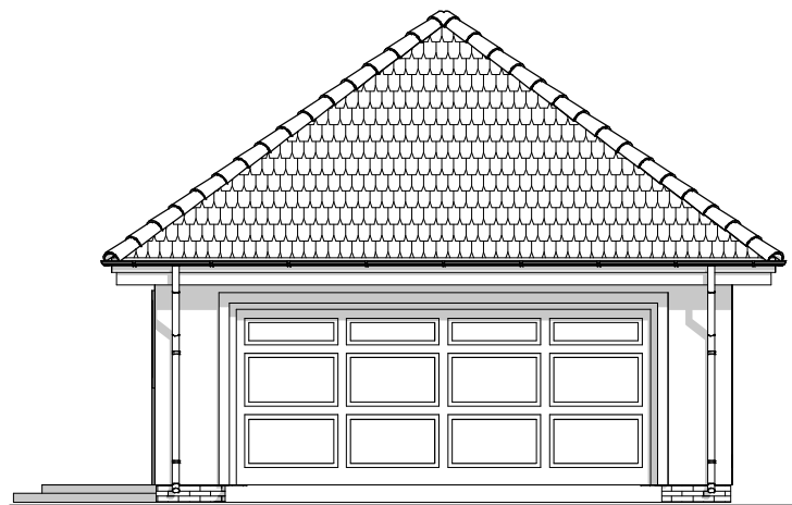
ELEWACJA FRONTOWA :
