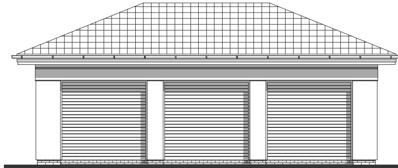
elewacja frontowa:
