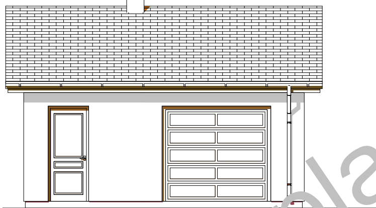
elewacja boczna :
