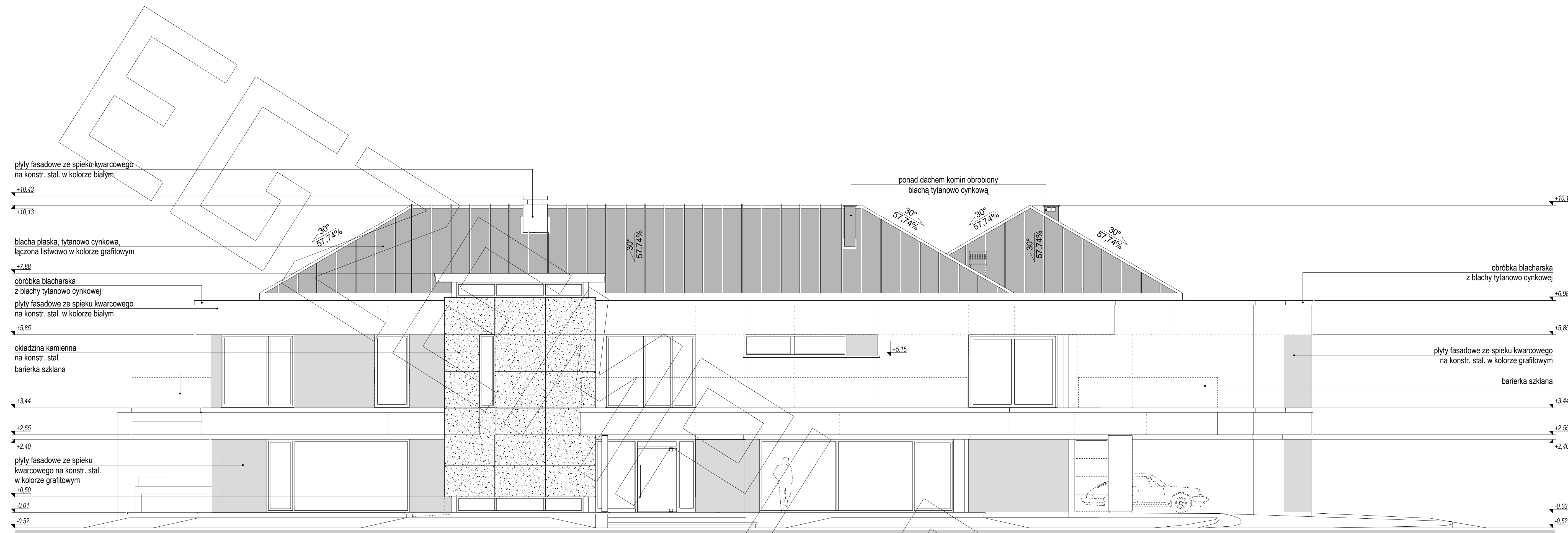
elewacja frontowa: wschodnia
