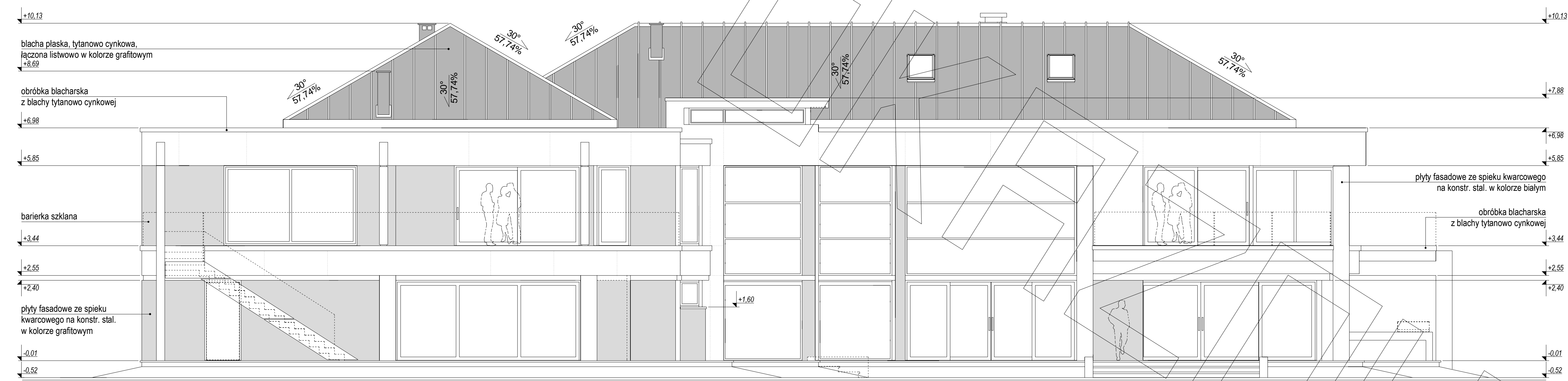
elewacja tylna: zachodnia
