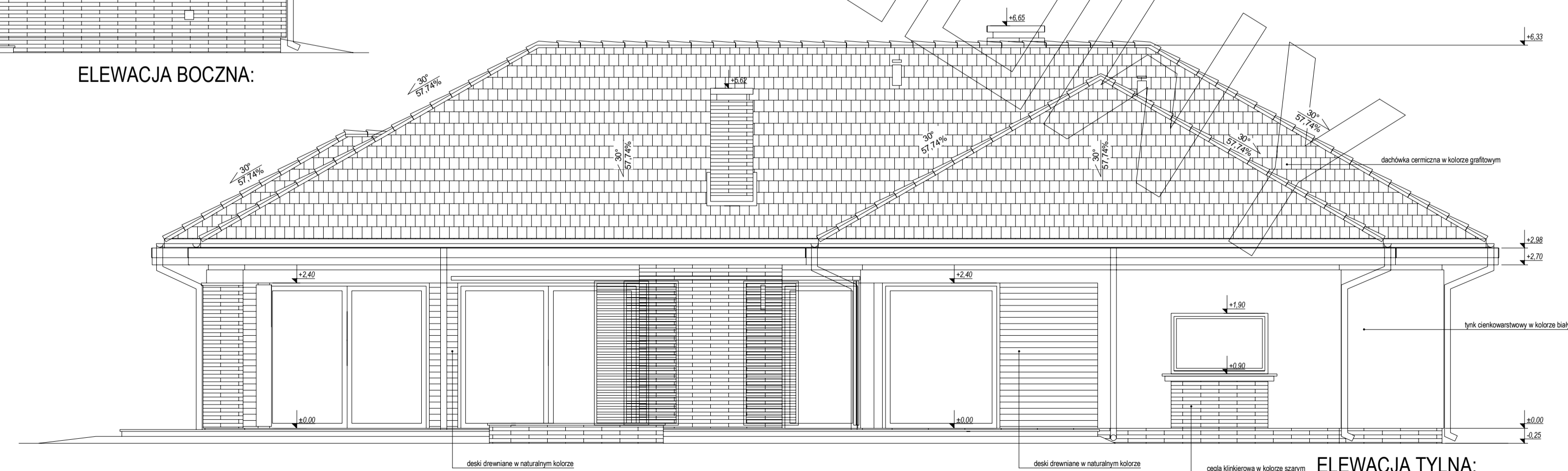
ELEWACJA TYLNA:
