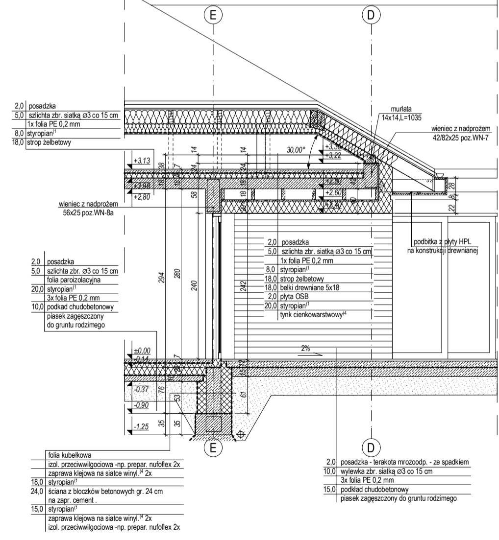
PRZEKRÓJ B3-B3
