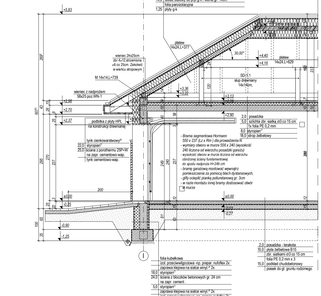
PRZEKRÓJ B1-B1
