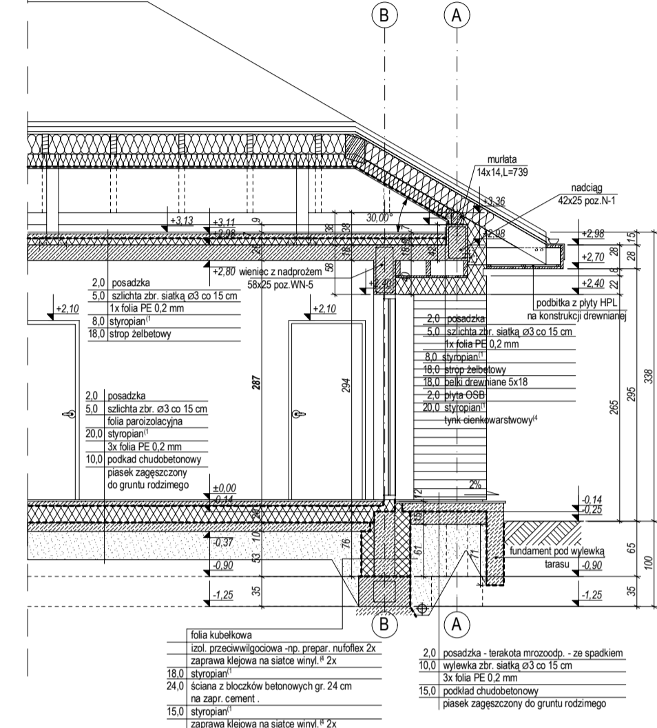
PRZEKRÓJ B2-B2
