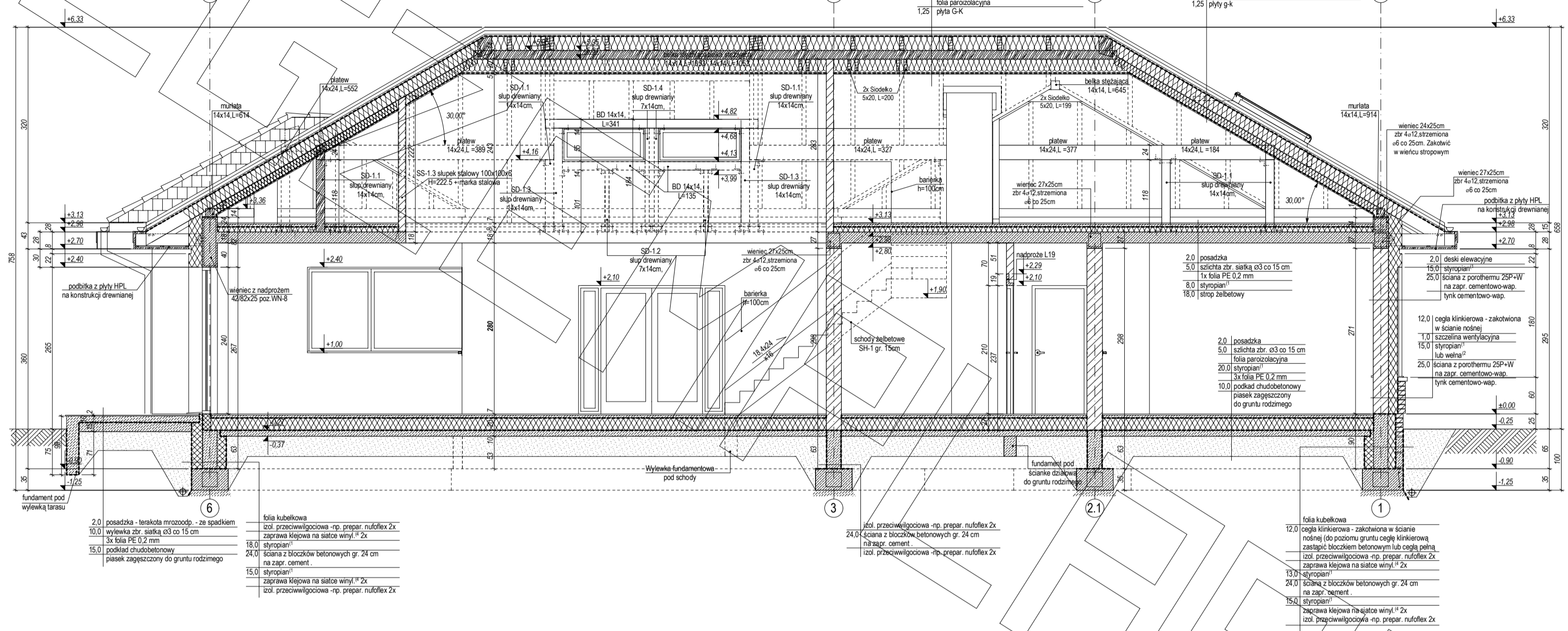
PRZEKRÓJ A-A
